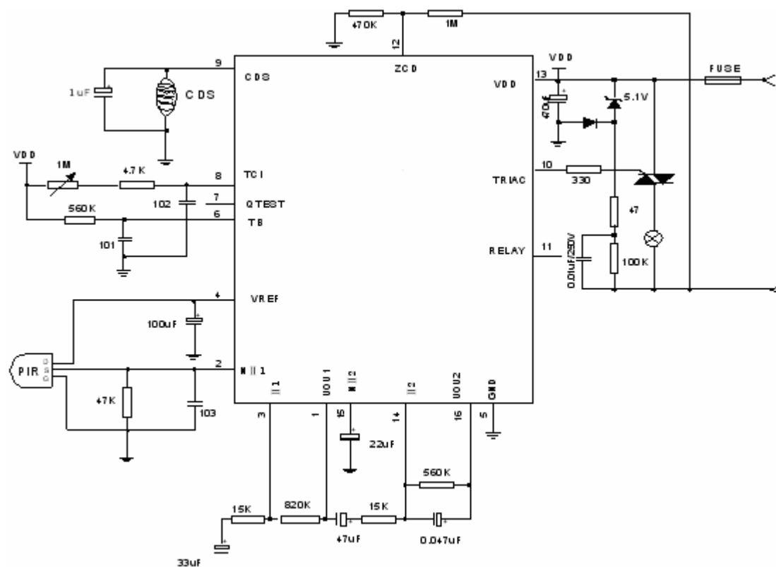
典型应用图 用于可控硅控制
